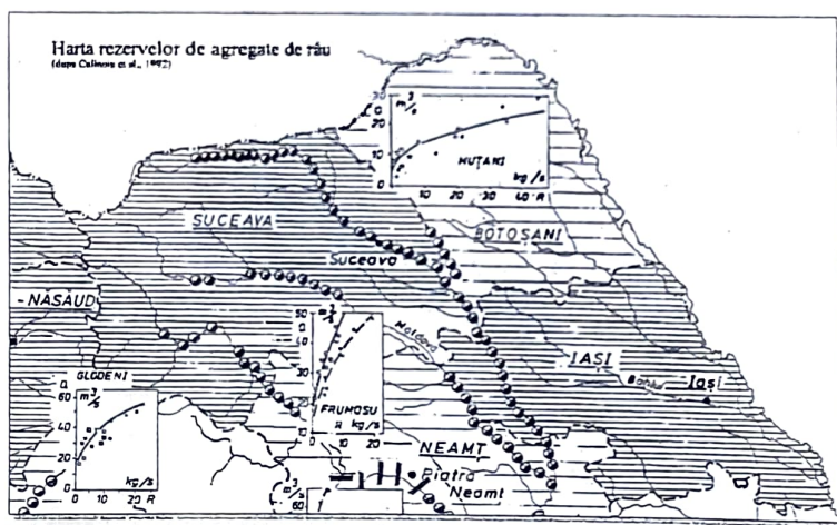
Fig. 1. Extras din harta rezervelor de agregate de râu (Călinoiu et al., 1988).
