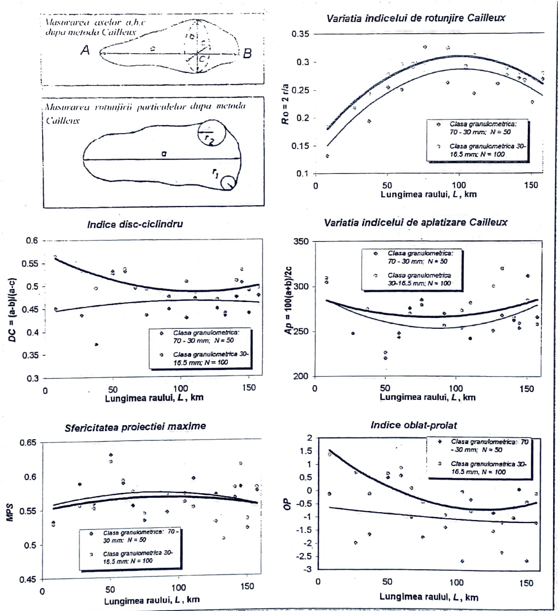
Fig. 7. Morfometria pietrișurilor din albia râului Suceava
