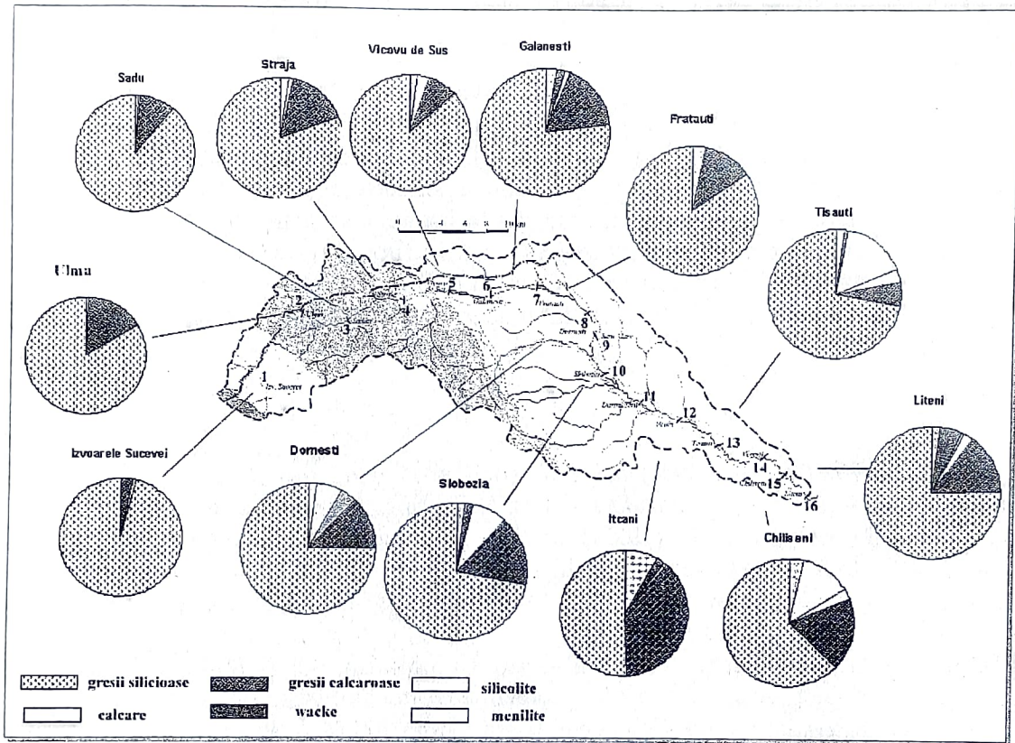
Fig. 10. Litologia pietrișurilor în lungul râului Suceava.
