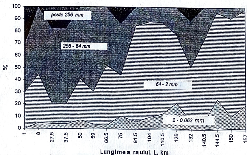
Fig. 4. Spectrul granulometric al depozitelor de albie ale râului Suceava.
