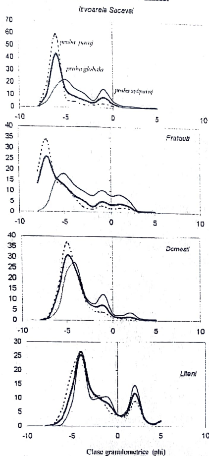
Fig. 6. Histogramele pentru secțiunile de probare în lungul râului Suceava care evidențiază fenomenul de bimodalitate.
