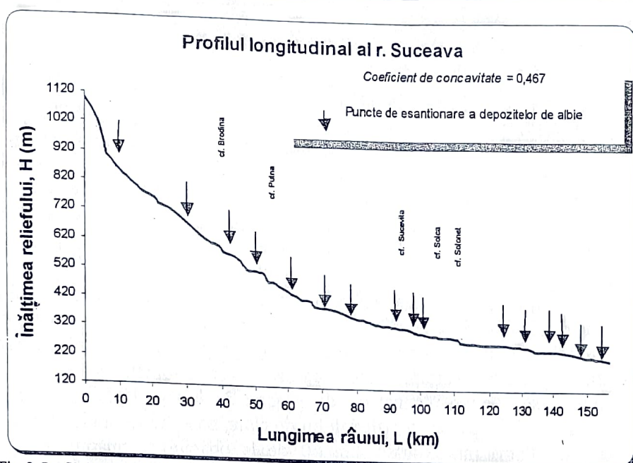
Fig. 3. Profilul longitudinal al râului Suceava, cu indicarea punctelor de eșantionare a materialului de albie.
