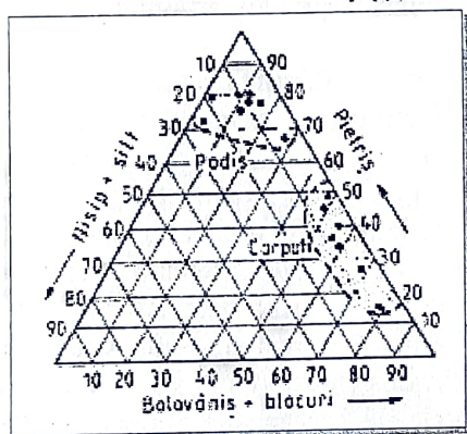
Fig. 5. Segregarea materialului de albie în lungul râului Suceava.
