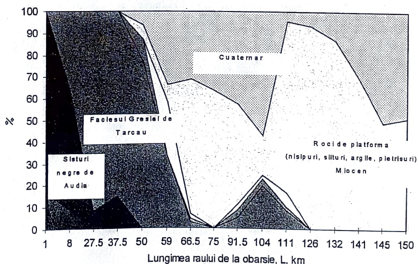
Fig. 8. Spectrul petrografic al bazinului hidrografic Suceava
