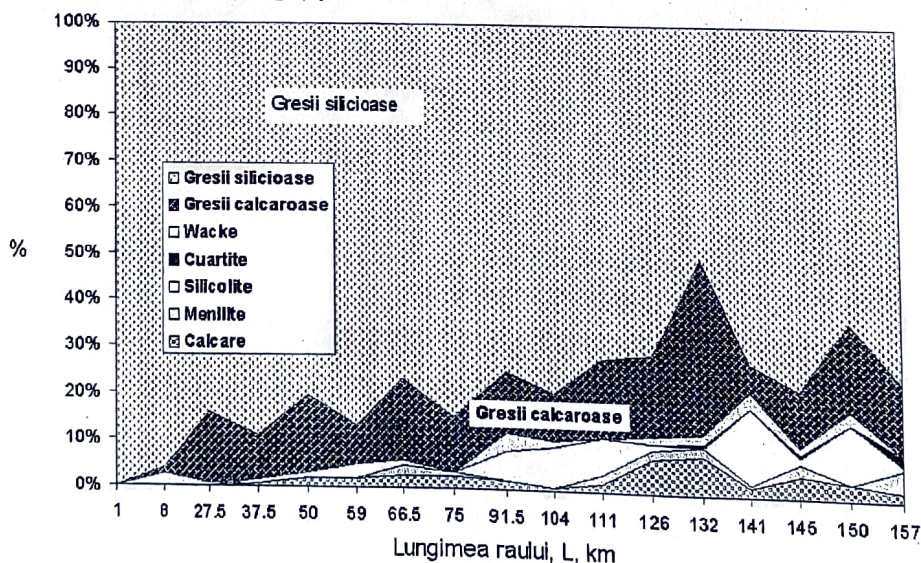
Fig. 9. Spectrul petrografic al pietrișurilor din albia râului Suceava.
